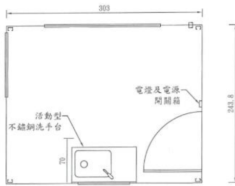
平面配置圖
